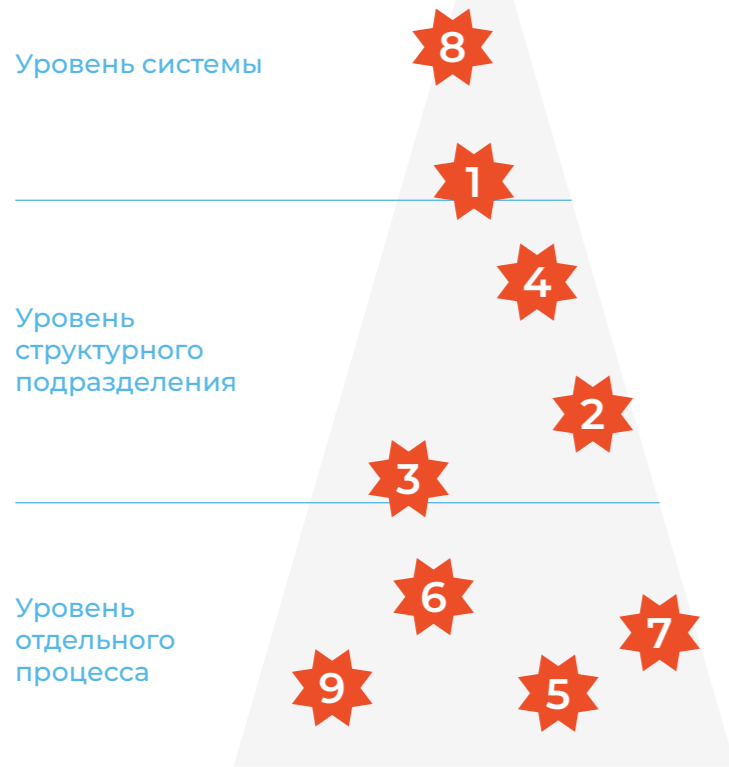
Рис. 5. Пирамида проблем
